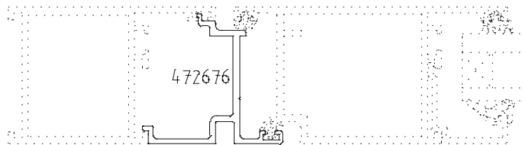
Einsatzprofil für nach außen öffnende Türen
