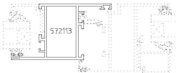
Sprossenprofil mit wechselndem Anschlag für wechselnde Verglasungsseiten
