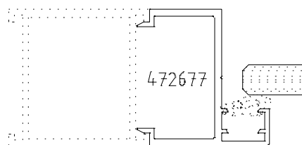
Einsatzprofil für Ganzglastüren
