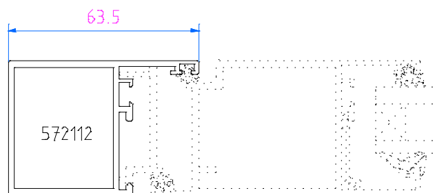
Blendrahmenprofil
