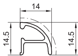
P 446618 Wetterschenkel
